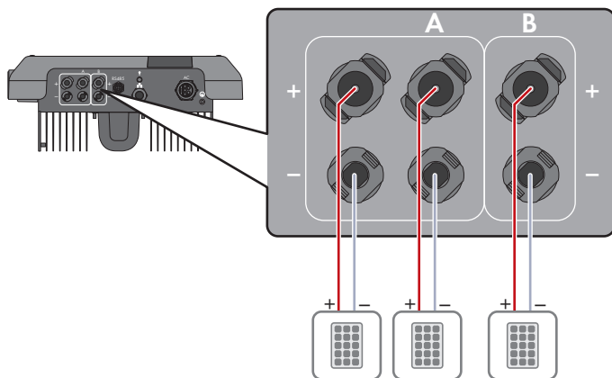
Figura 10: Privire de ansamblu asupra conexiunii în modul de funcționare normal
