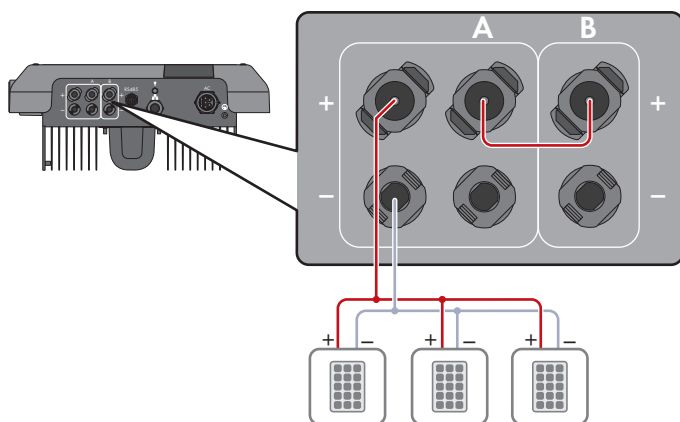
Figura 11: Privire de ansamblu asupra conexiunii la conectarea în paralel a intrărilor DC A și B
