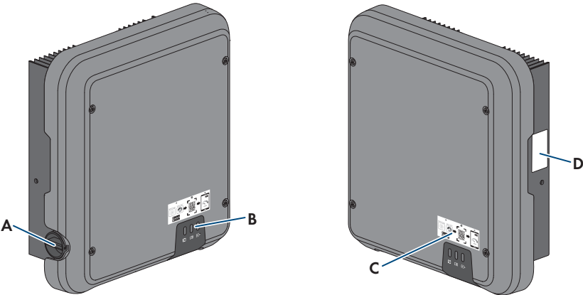
Figura 2: Structura produsului
